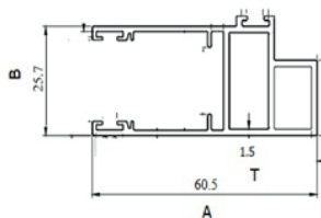
PSPMOS01 MOSQUITO SHUTTER SERIES(MOS)
