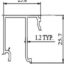
PSP3610 CASEMENT CLIP
