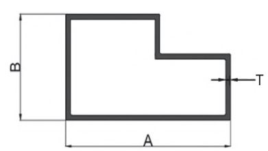
PSP1181 SIMPLE L-TUBE
