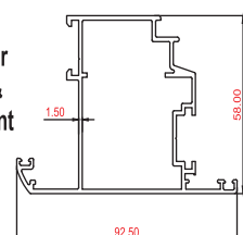
PSP5024 50mm Door Shutter
