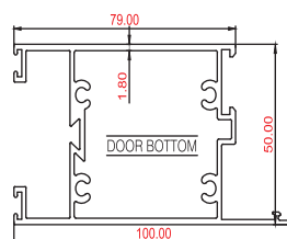
PSP5026 50mm Door Bottom
