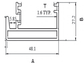
PSP3612 36MM SLEEK INTERLOCK
